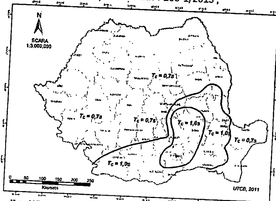
Figura A.2 Zonarea teritoriului României în termeni de perioadă de control (colt), T_C a spectrului de răspuns
