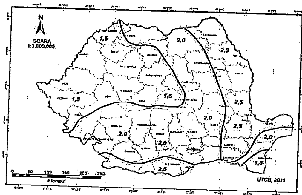
Figura 3.1 Zonarea valorilor caracteristice ale incarcarii din zapada pe sol s_0, kN/m^2 , pentru altitudini A = 1000 \text{ m} NOTA: Pentru altitudini A > 1000 \text{ m} valorile s_0 se determina cu relatia (3.1) si (3.2)
