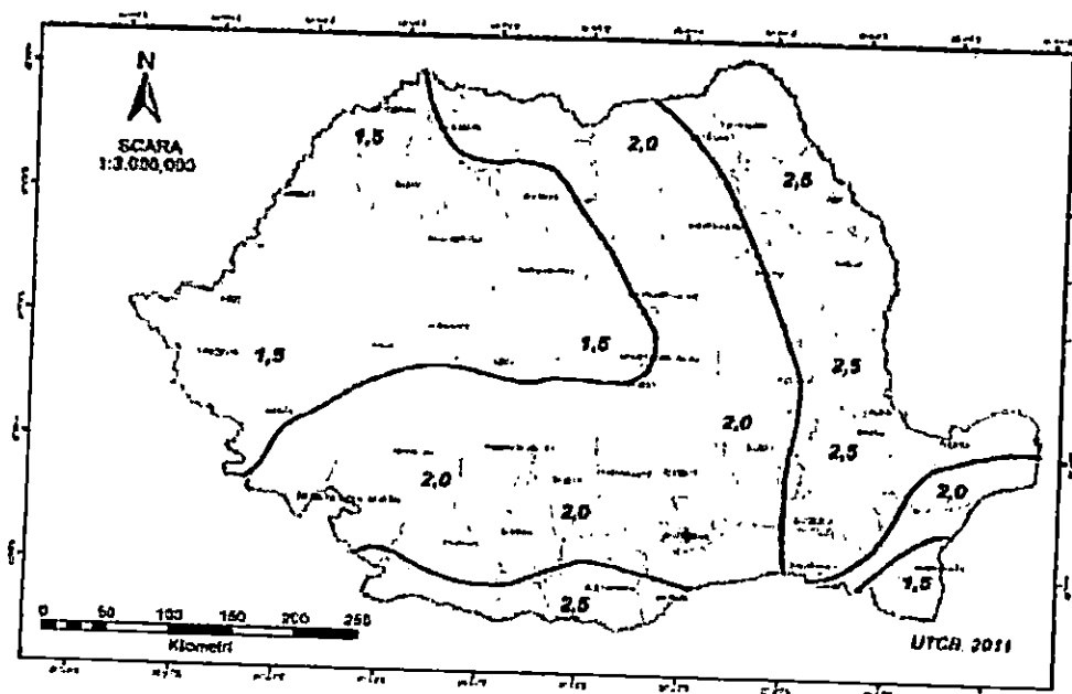
Figura 3.1 Zonarea valorilor caracteristice ale incarcarii din zapada pe sol s_{0,k} , \text{kN/m}^2 , pentru altitudini A = 1000 \text{ m} NOTA: Pentru altitudini A > 1000 \text{ m} valoarea s_{0,k} se determina cu relatia (3.1) si (3.2)
