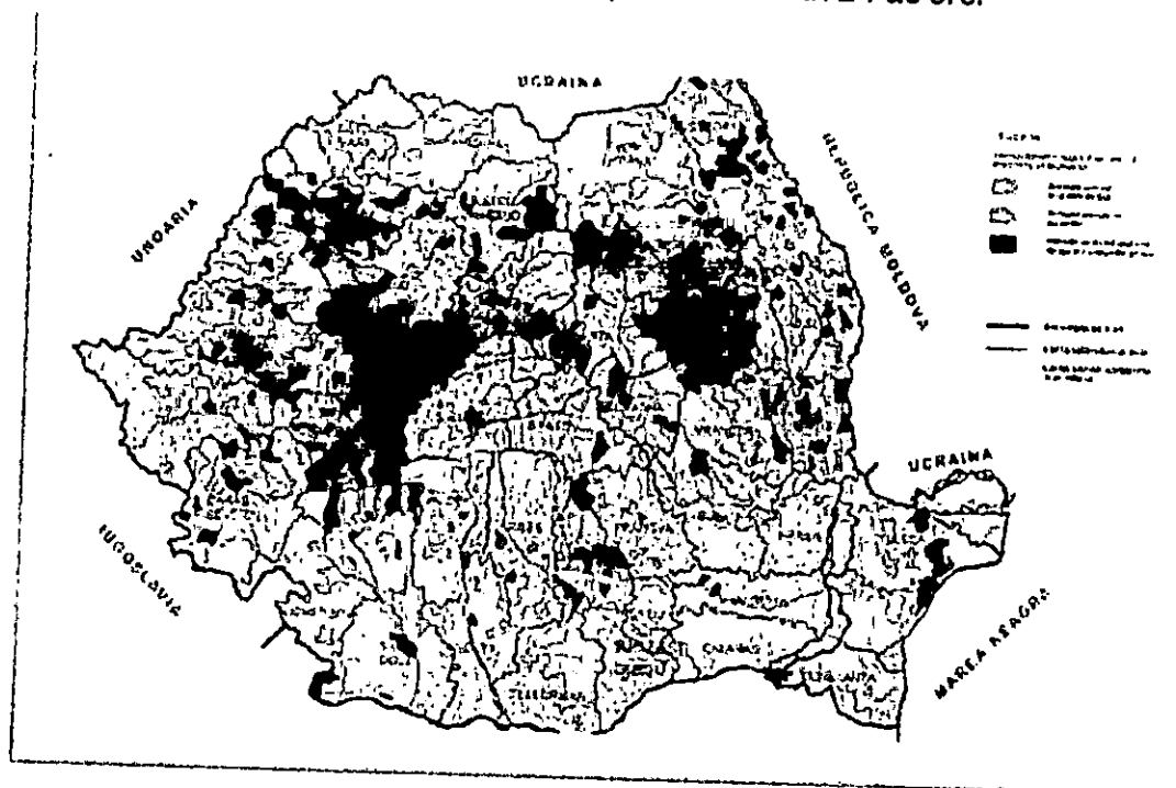
Planul de Amenajare a Teritoriului National – Sectiunea a V-a – Zone de risc natural: Tipuri de inundatii
