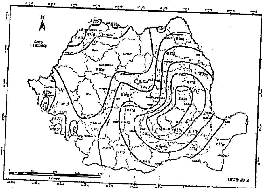
Figura A.1 România - Distribuția valorilor de vârf ale accelerației terenului pentru proiectare a_g cu IMR = 225 ani și 20% probabilitate de depășire în 50 de ani
