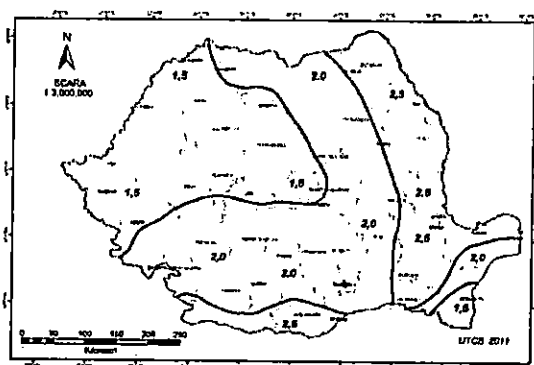
Figura 3.1 Zonarea valorilor caracteristice ale încărcării din zapada pe sol s_k , kN/m^2 , pentru altitudin A \leq 1000 m
