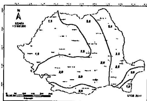
Figura 3.1 Zona de valori caracteristice ale încărcării din zapada pe sol s_k , kN/m 2 , pentru altitudinile A \leq 1000 m
