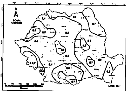
Figura 3.2 Zona de valori de referință ale presiunii dinamice a vântului, în kPa, pentru altitudinile A \leq 1000 m
